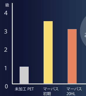
■ 汚れ除去性 (ダイヤモンド法)
