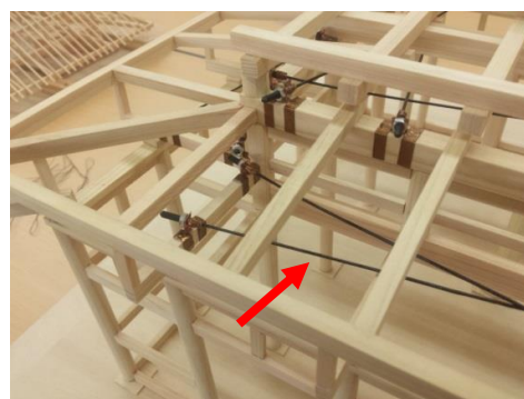
カボコーマ・ストランドロッドによる施工（イメージ）
