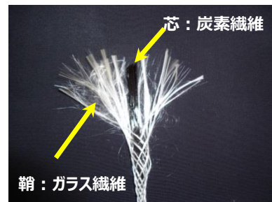
ロッドの構造
